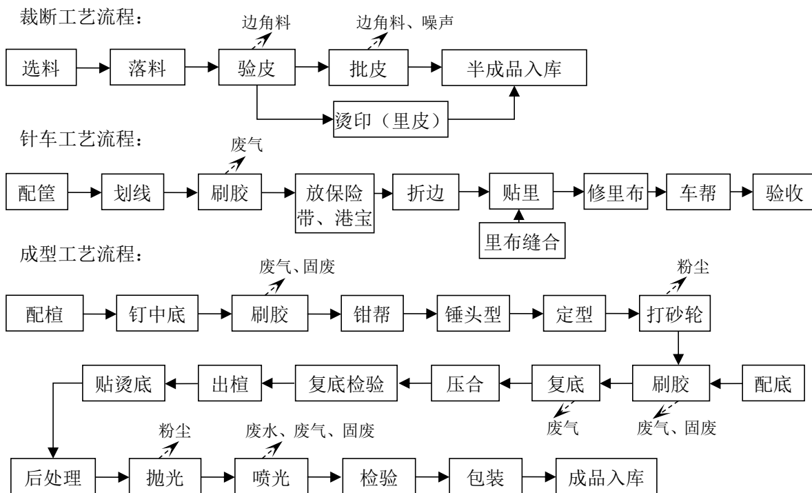
图 3-4 项目工艺流程图及产污环节图
